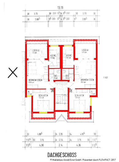
Grundriss Dachgeschoss
