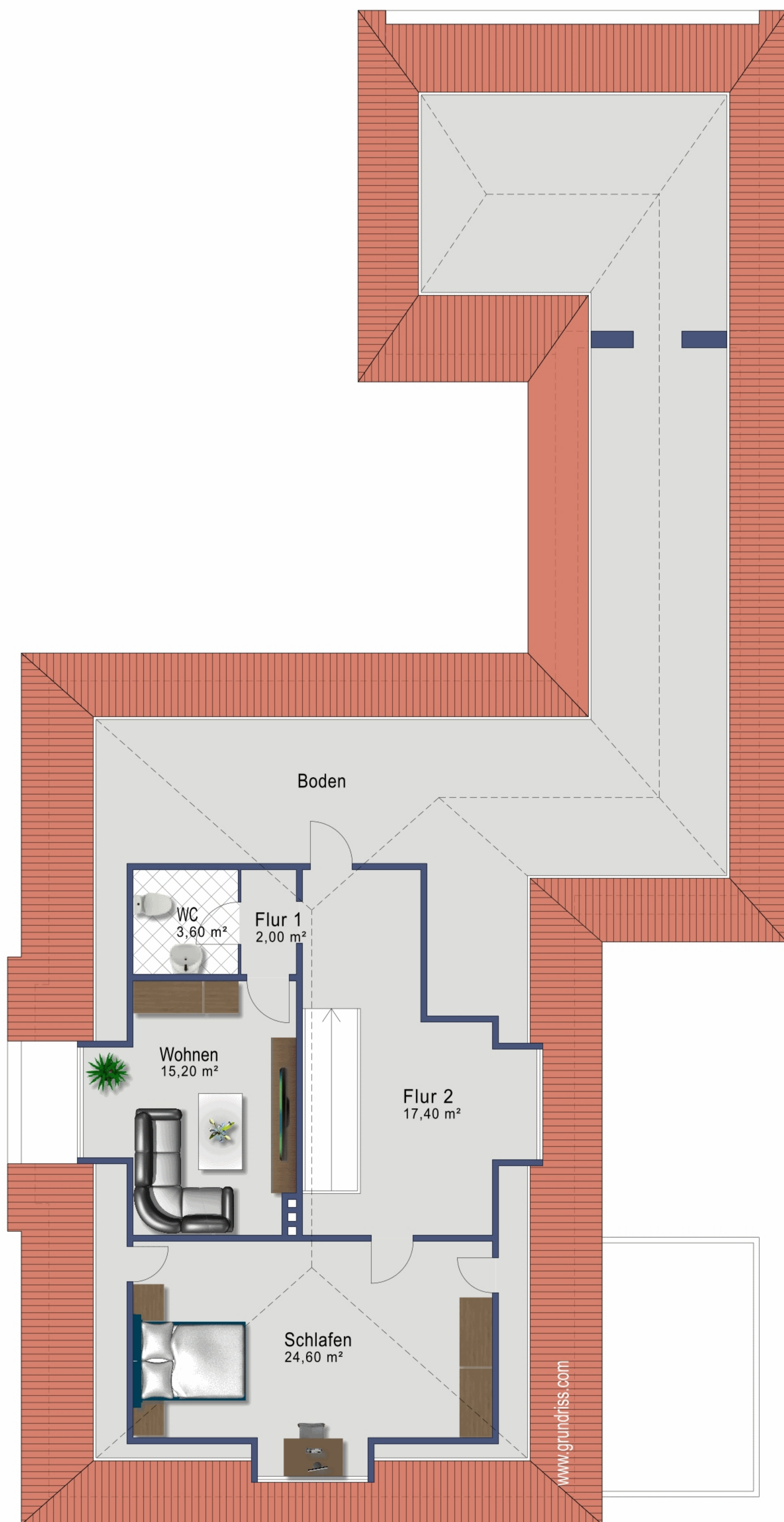
Dachgeschoss
