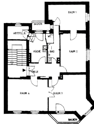
Grundriss
