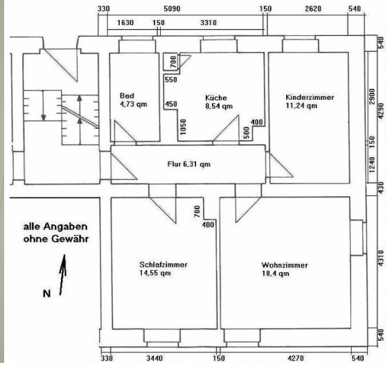
Grundriss
