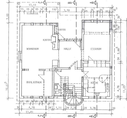
Grundriss Erdgeschoss
