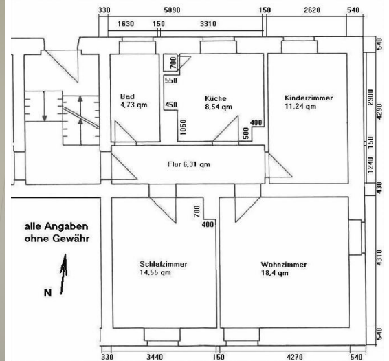
Grundriss
