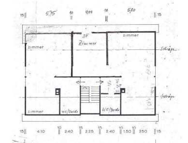
Grundriss DG
