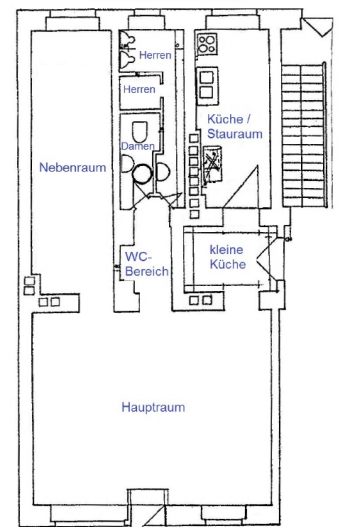
Grundriss Bar
