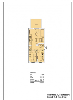
Grundriss
