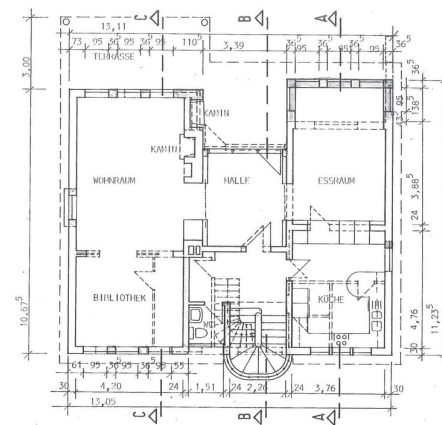
Grundriss Erdgeschoss
