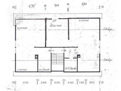
Grundriss DG
