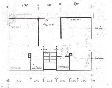
Grundriss DG
