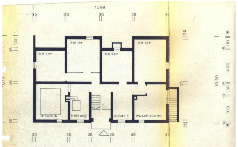
Grundriss KG
